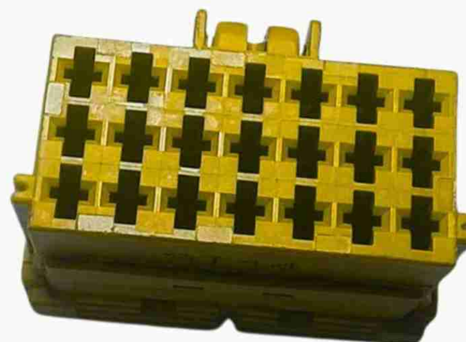
COD: D2020-21-AM Conector 021 VIAS
