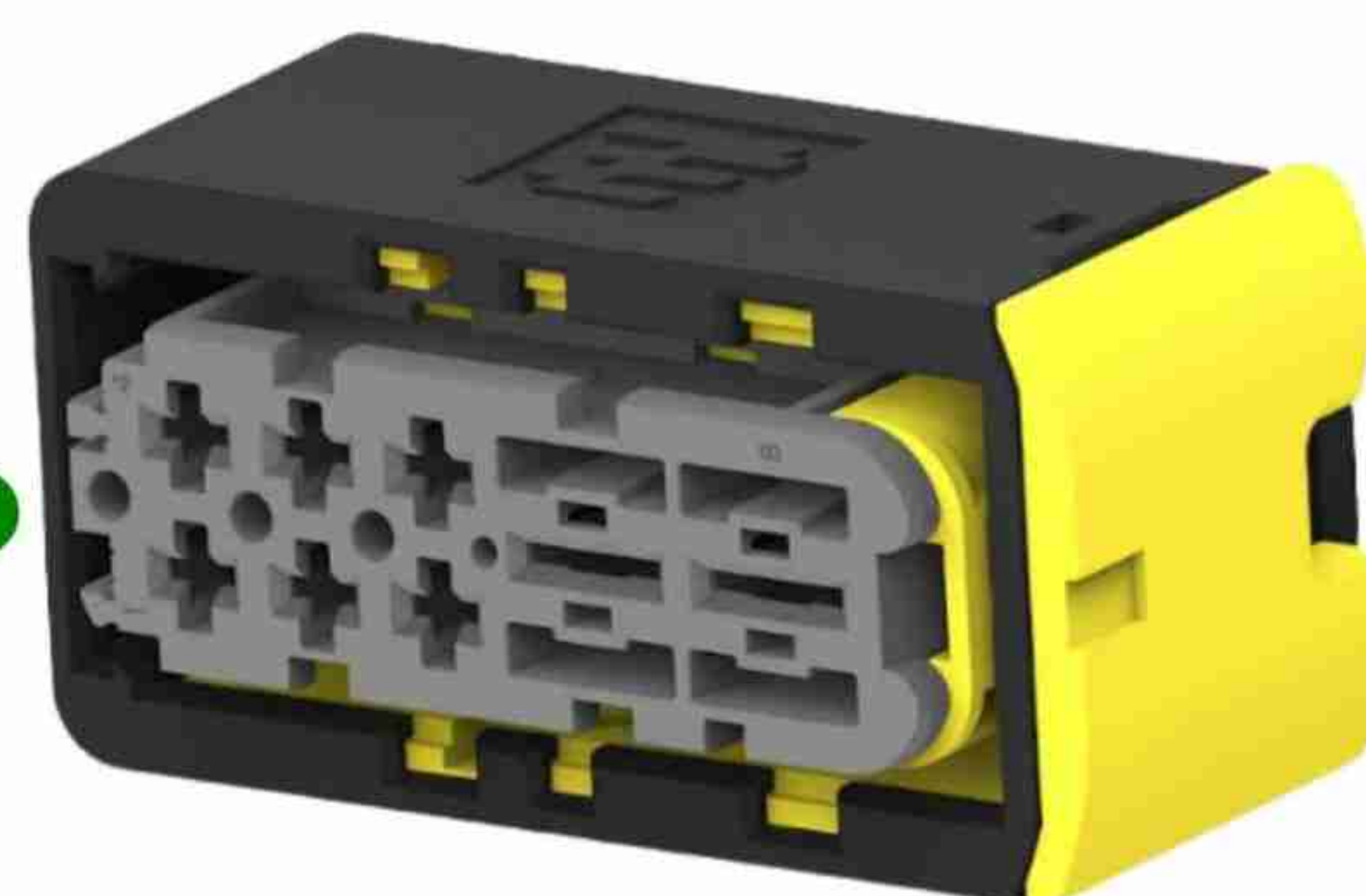
COD: D2130-C Conector 006 VIAS
