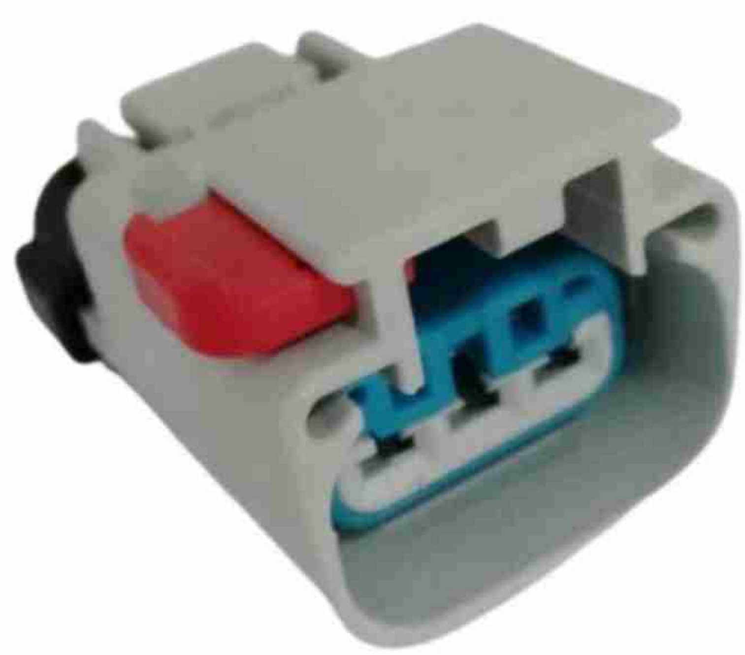
COD: 03.0036-B Conector 003 VIAS
