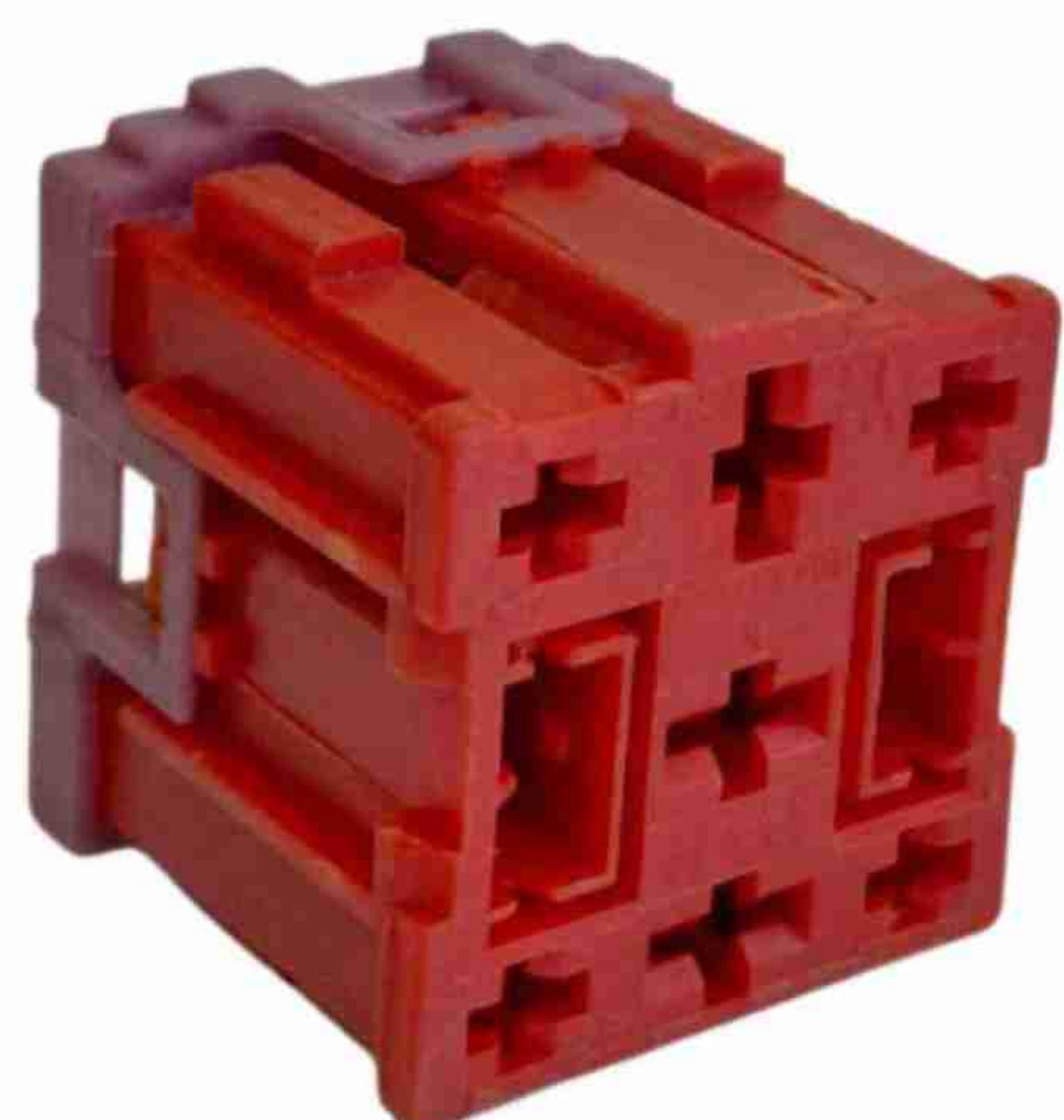
COD: 09.0001 - VERMELHO Conector 009 VIAS
