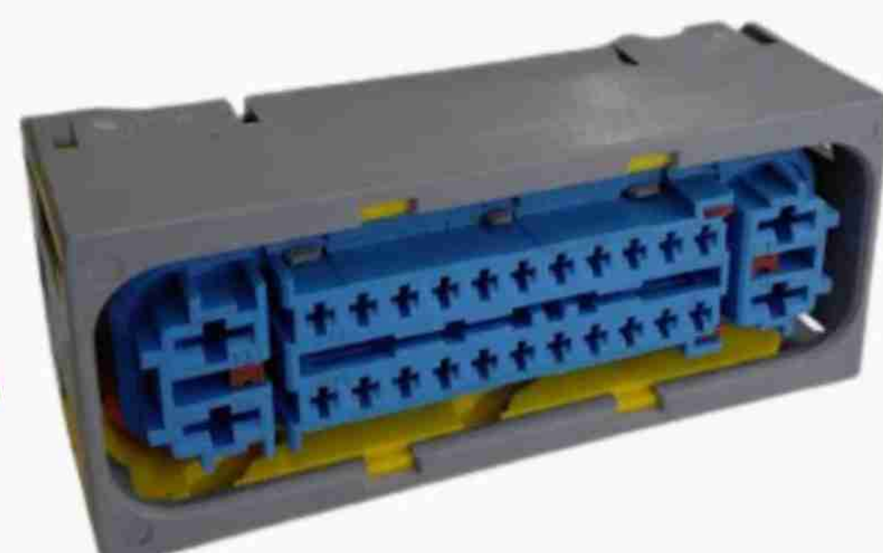
COD: 19.0003 Conector 019 VIAS
