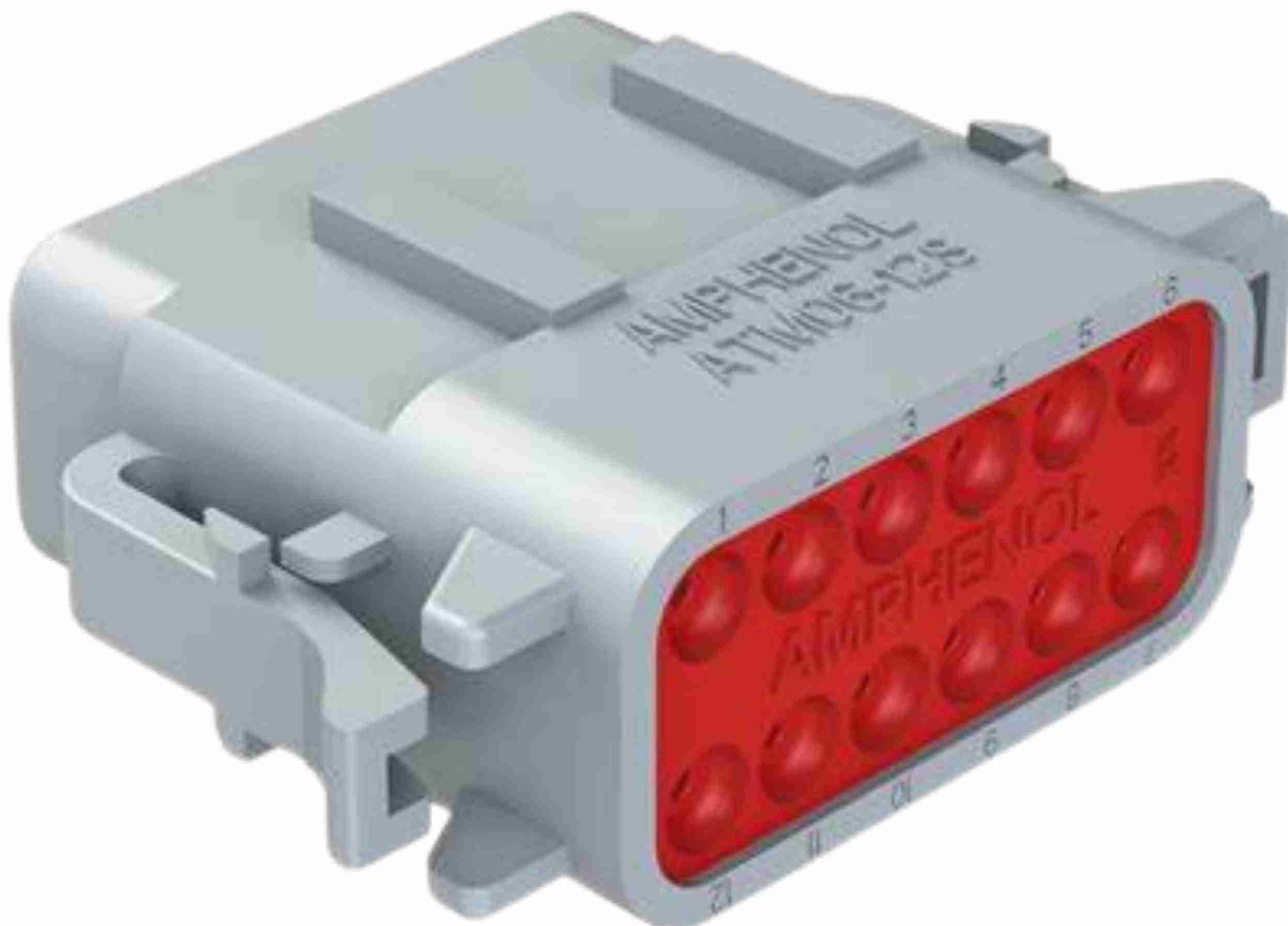
COD: AT06-12SA Conector 012 Vias
