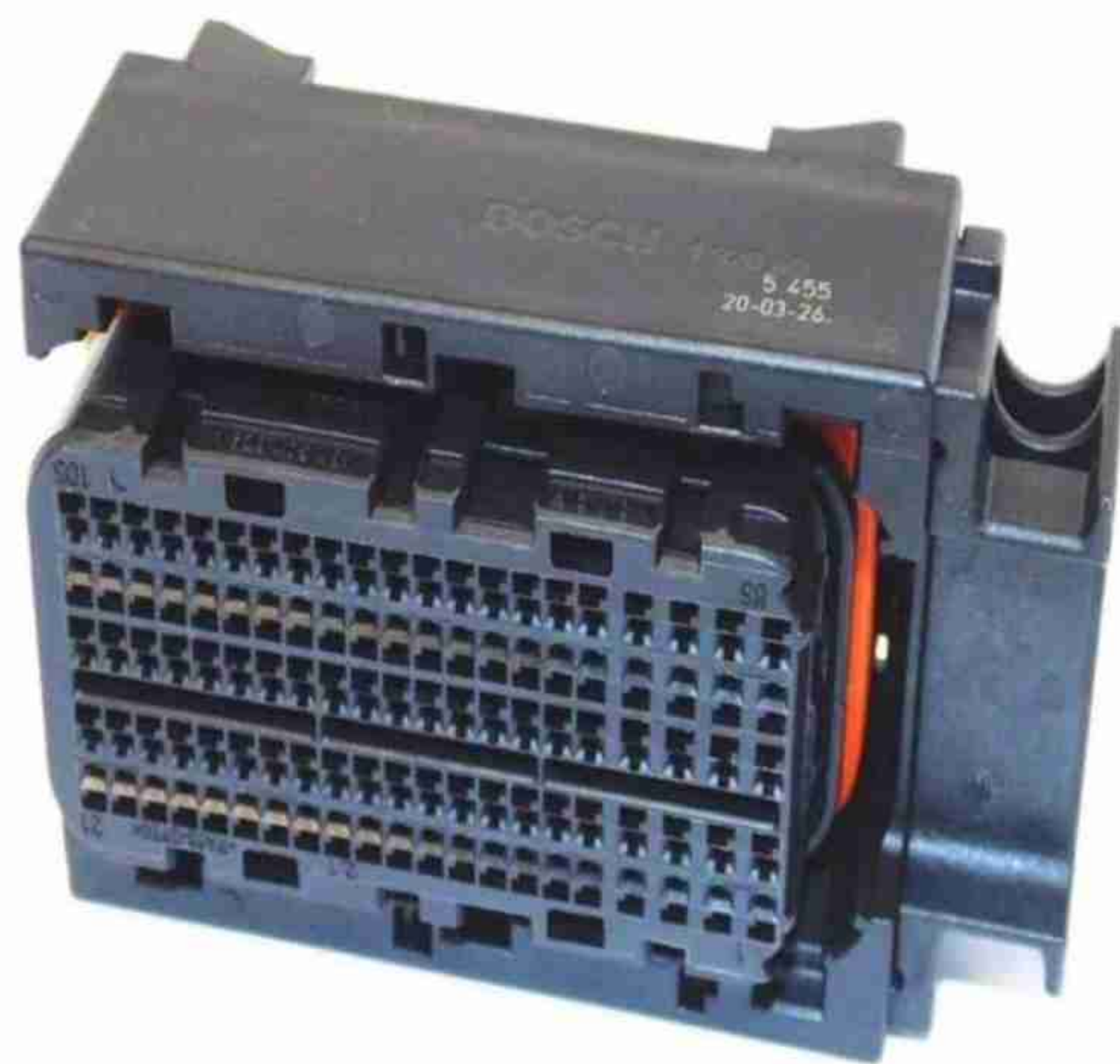
COD: 105.0002 Conector 105 VIAS
