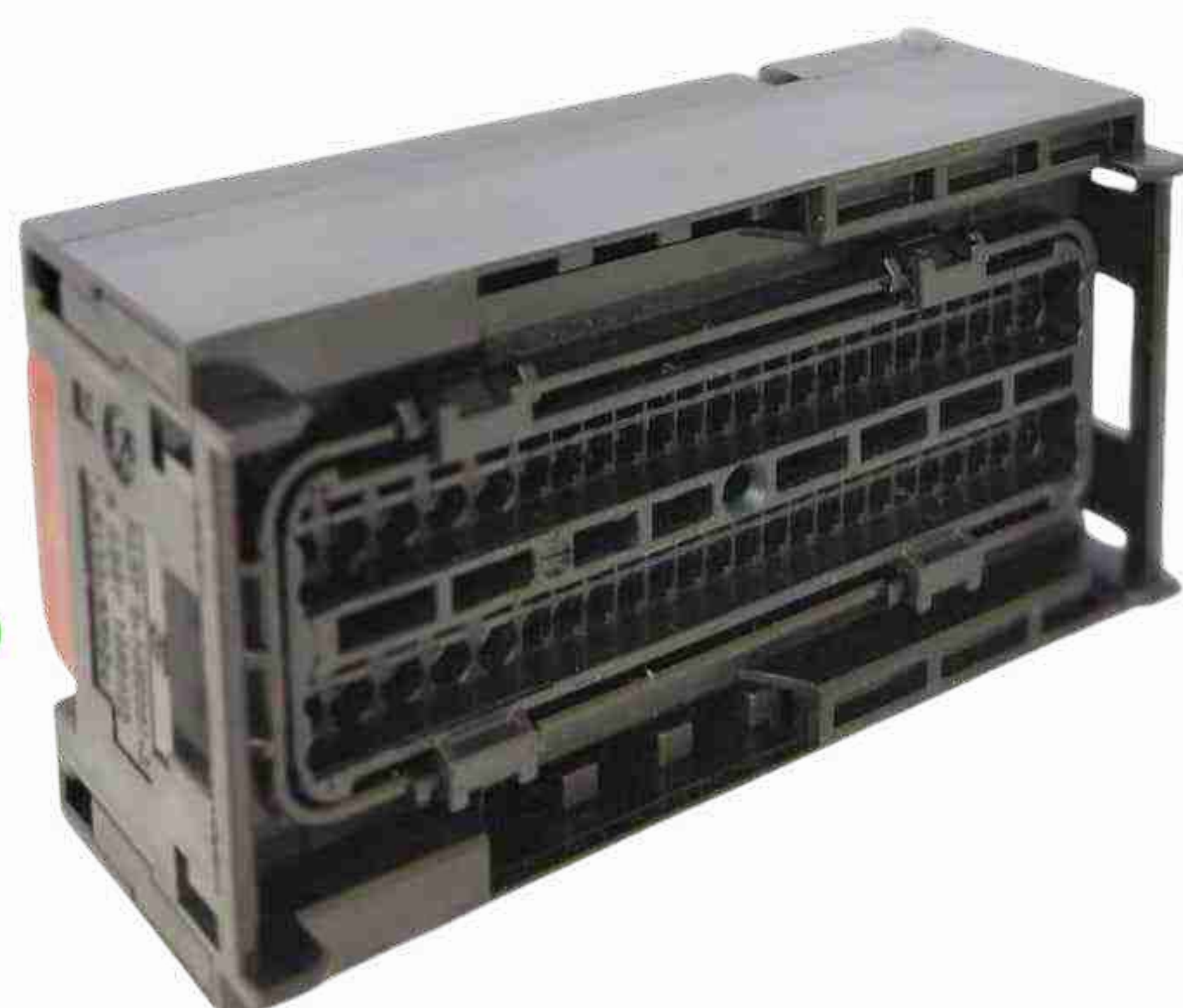
COD: 96.0005 Conector 096 VIAS
