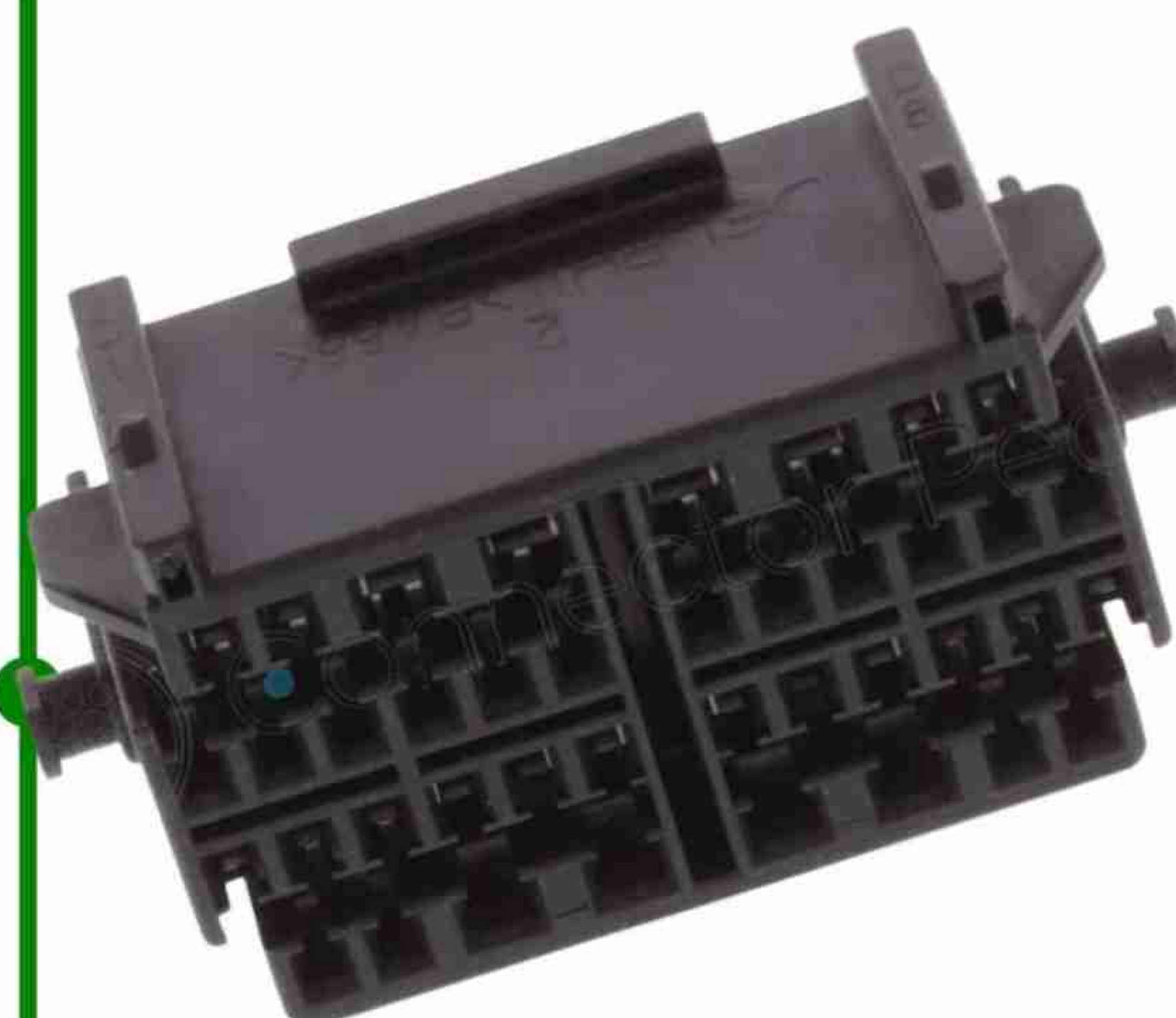
COD: 40.0001 Conector 040 VIAS
